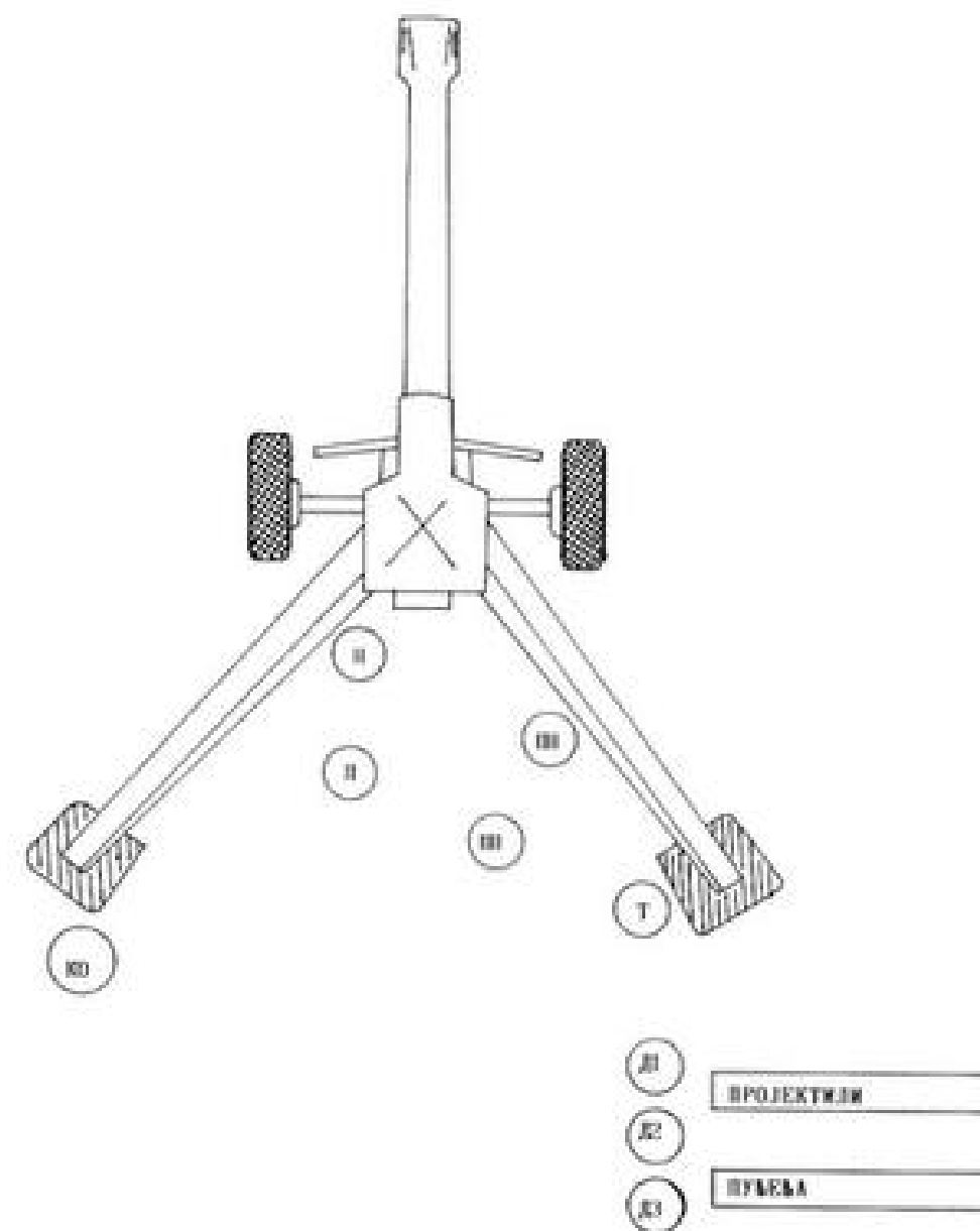
Слика број 46 б – Место послуживоца код оруђа кад је оруђе у положају спремно за паљбу
