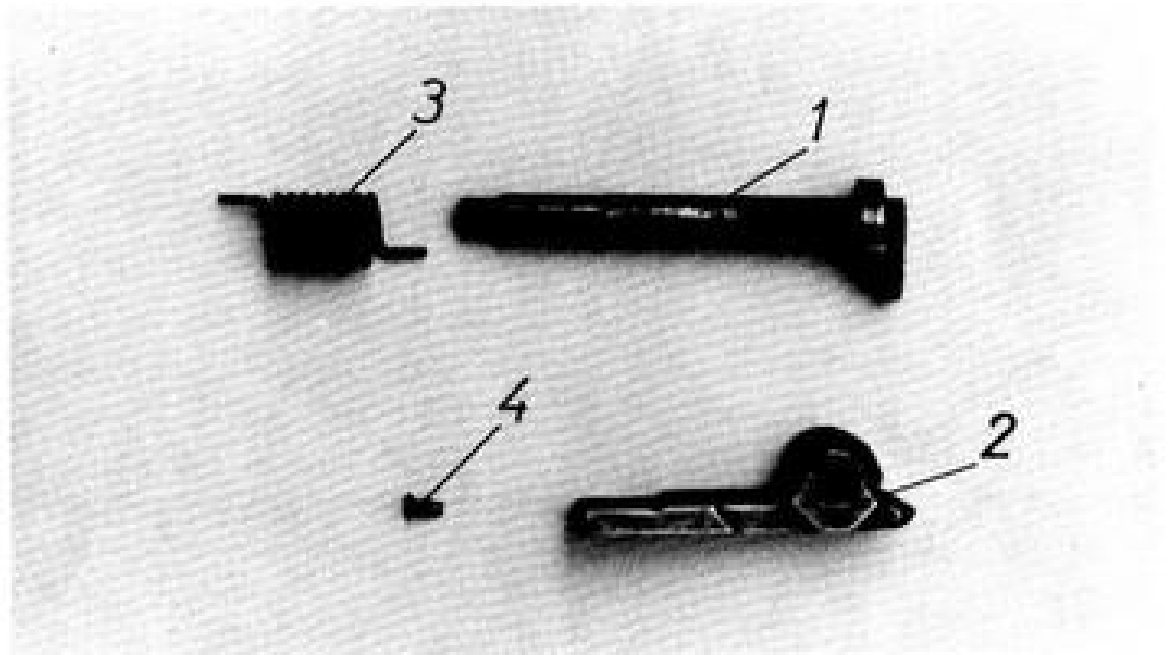
Слика број 12 а – Група делова за задржавање пројектила 1. – Осовина задржача, 2. – Задржач пројектила, 3. – Опруга, 4. – Вијак утврђивача
