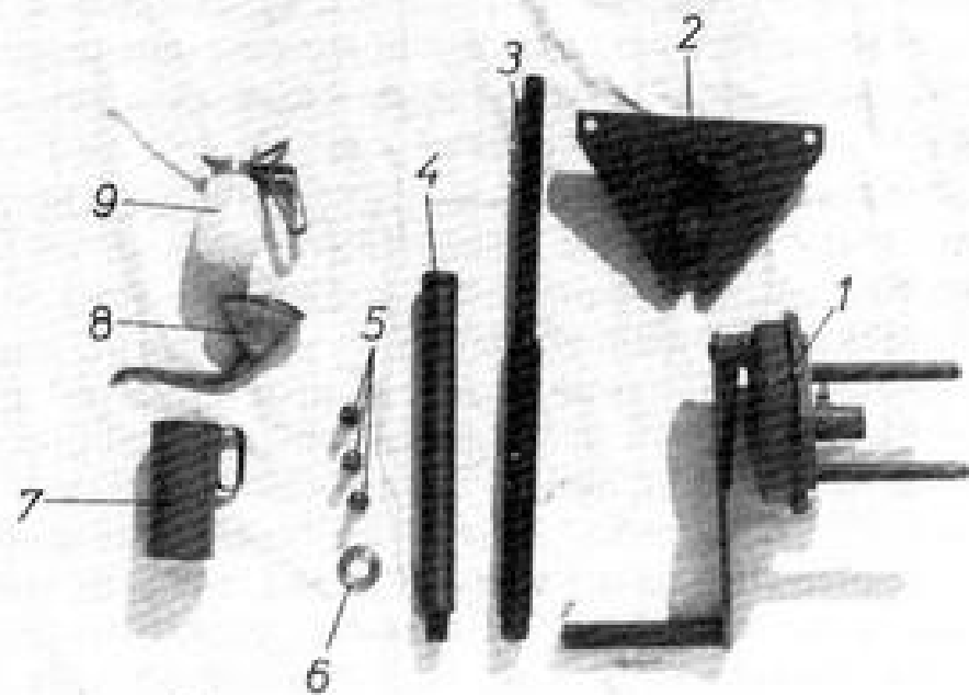
Слика број 44 – Уређај за вентилско трљање цеви
