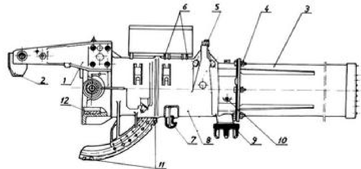
Слика број 16 – Колевка
