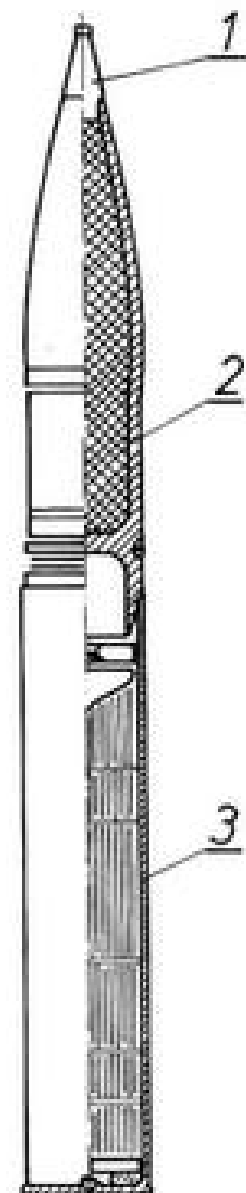
Слика број 48 б – Метак са ТФ пројектилом 152 mm М84 1. – Упаљач, 2. – ТФ пројектил 152 М84, 3. – Чаура са топовском капслом
