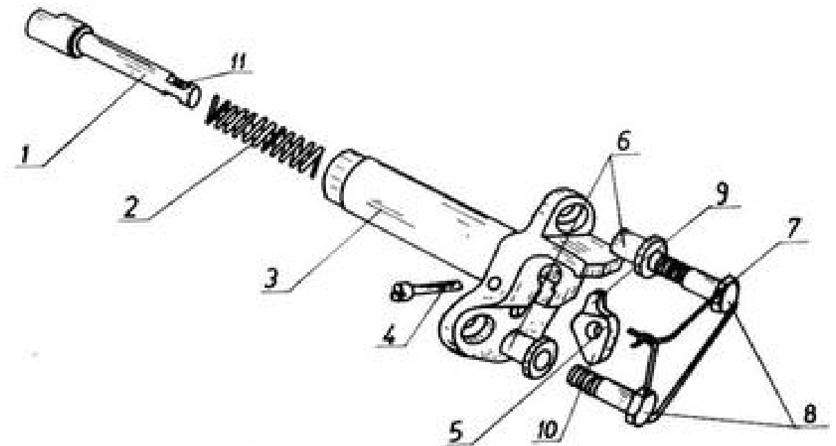
Слика број 13 – Делови за блокирање механизма за затварање затварача 1. – Утврђивач, 2. – Опруга, 3. – Ослонац ручице, 4. – Осовина полуге, 5. – Двокрака полука, 6. – Чаура, 7. – Жица за осигурање, 8. – Вијци, 9. – Горњи крак двокраке полуге, 10. – Доњи крак двокраке полуге, 11. – Прорез
