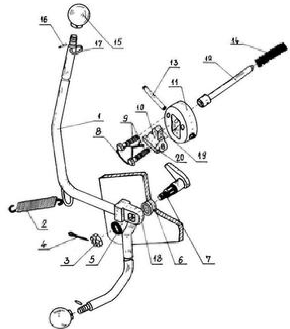
Слика број 8 ц – Ручица за окidaње са обарачом
