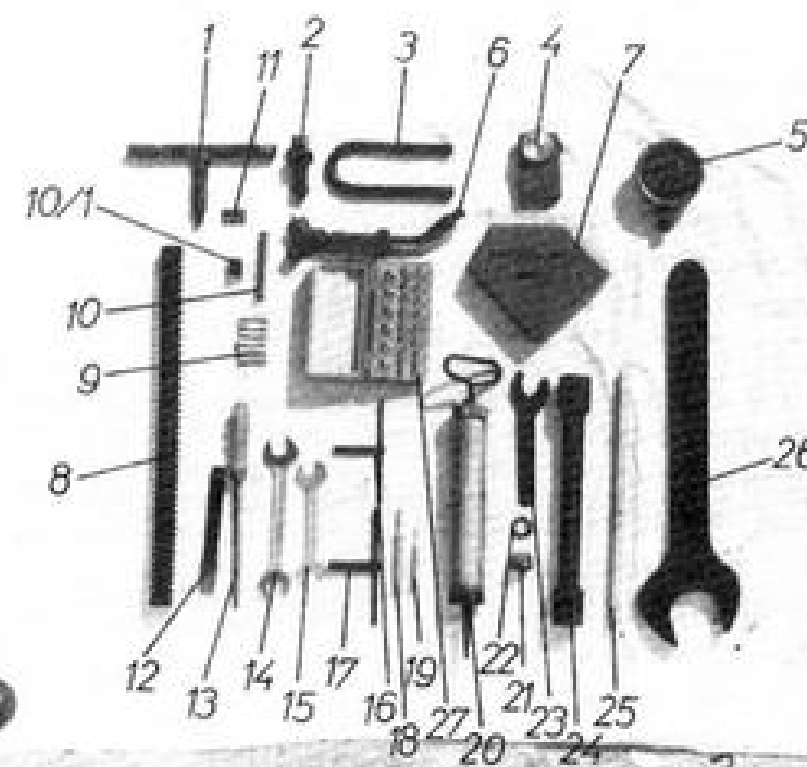
Слика број 42 – Батеријски РАП
