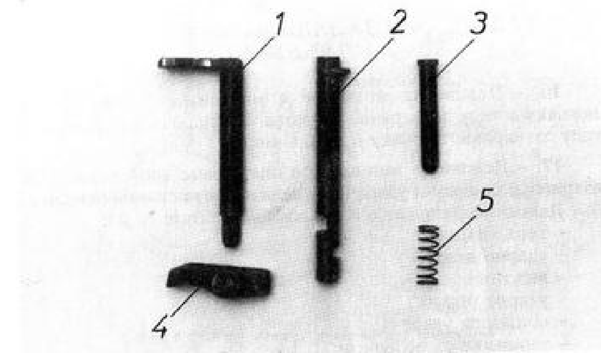
Слика број 8 б – Делови за затварање
