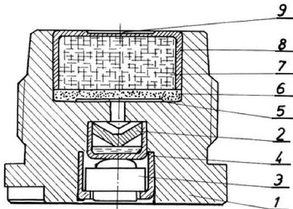
Слика број 56 – Тоновска капсула ТК-М71
