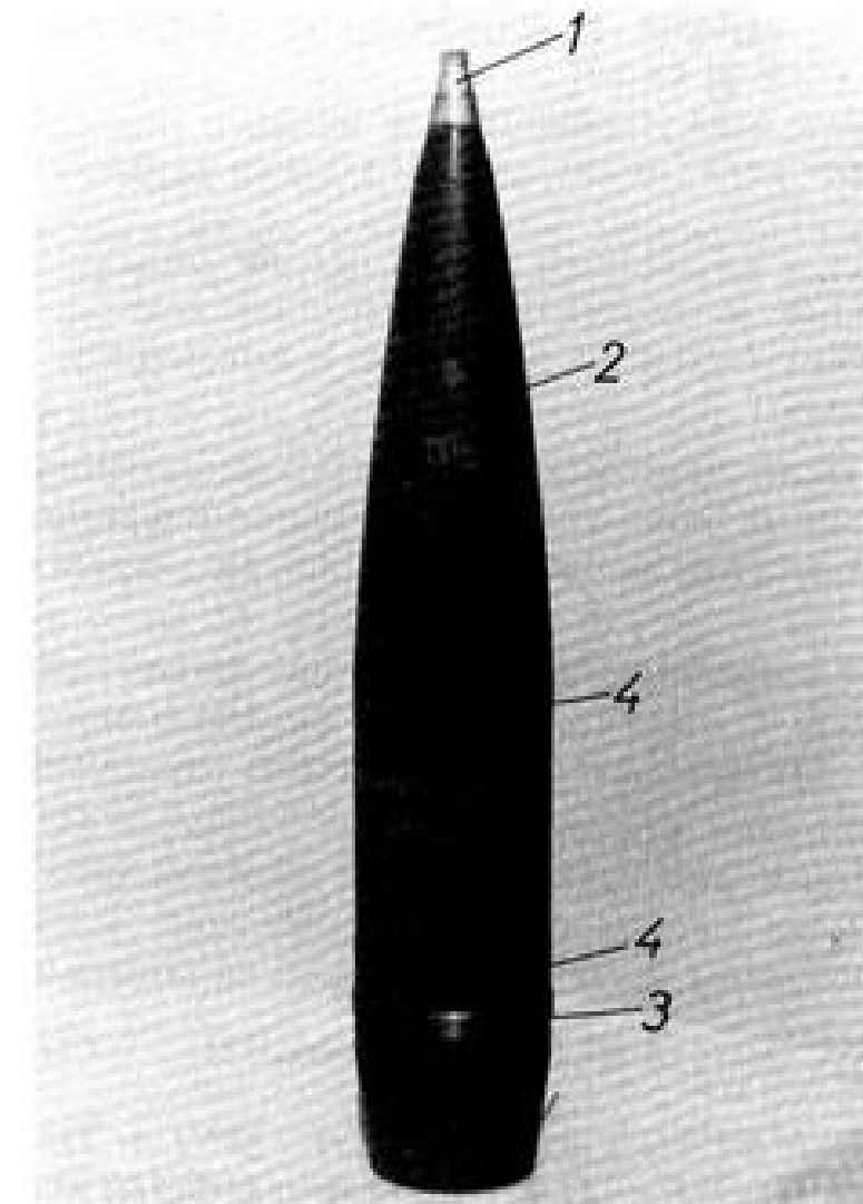
Слика број 48 а – ТФ пројектил 152 mm М-84 са упаљачем 1. – Упаљач, 2. – Кошуљица, 3. – Водећи прстен, 4. – Центрирајући прстен.
