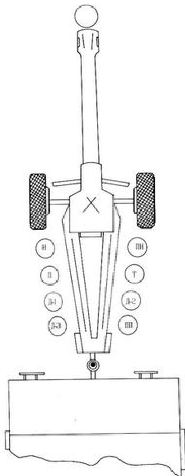
Слика број 46 а – Место послуживоца код оруђа кад је оруђе у положају спреман за мари
