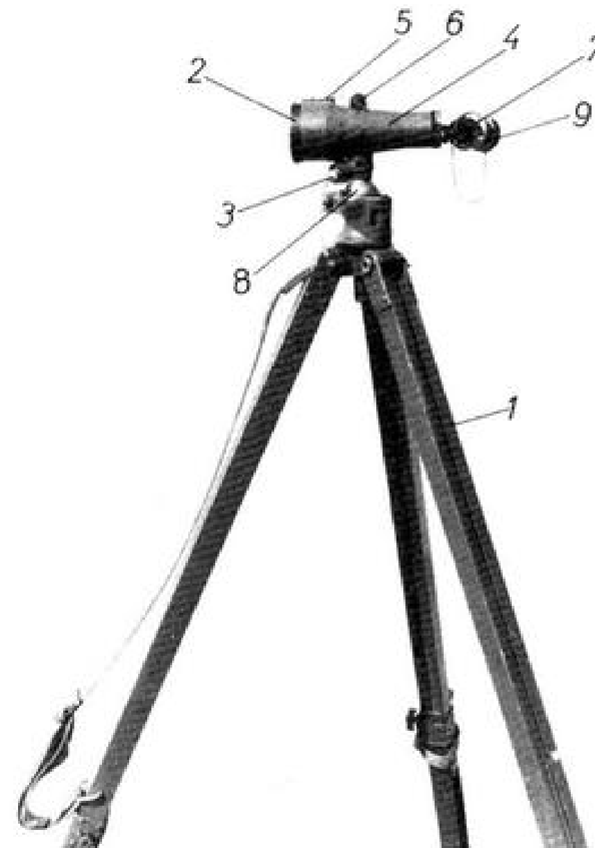
Слика број 36 – Колиматор К-М78
