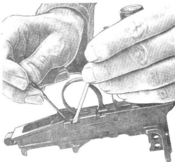
Sl. 78 - Isključivanje oslonca opruge poluge iz zahvata sa utvrđivačem
