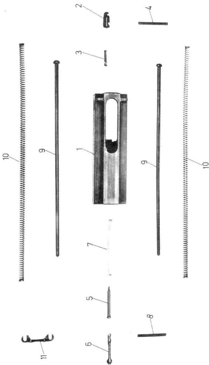
Sl. 35 - Delovi sklopa zatvarača sa opružnim povratnikom: 1 - zatvarač; 2 - izvlakač; 3 - opruga izvlakača; 4 - osovina izvlakača; 5 - udarna igla-prednji deo; 6 - udarna igla-zadnji deo; 7 - opruga zadnjeg dela udarne igle; 8 - osovina zadnjeg dela udarne igle; 9 - vodica povratne opruge; 10 - povratna opruga; 11 - utvrđivač povratne opruge.
