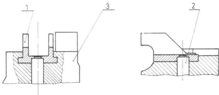
Sl. 13 - Izbačaj i njegova veza sa usadnikom:
