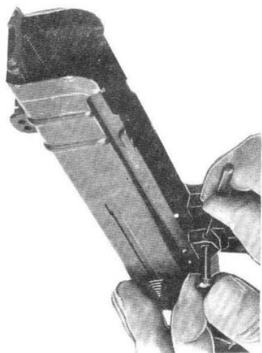
Sl. 56 – Odvajanje vodice zatvarača od usadnika
