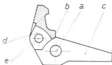
Sl. 24 – Zub obarače:
