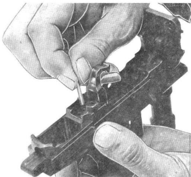
Sl. 74 – Odvajanje utrdne osovine izbacaja
