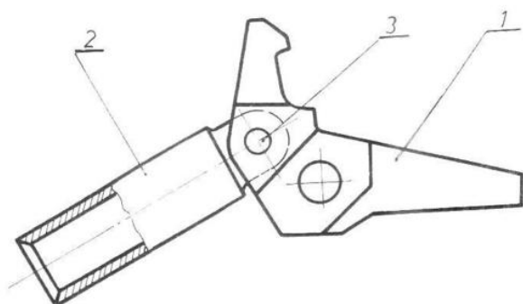
Sl. 23 – Zub obarače–ned. spoj: 1 – zub obarače; 2 – vođica udarne opruge; 3 – osovina vođice udarne opruge.
