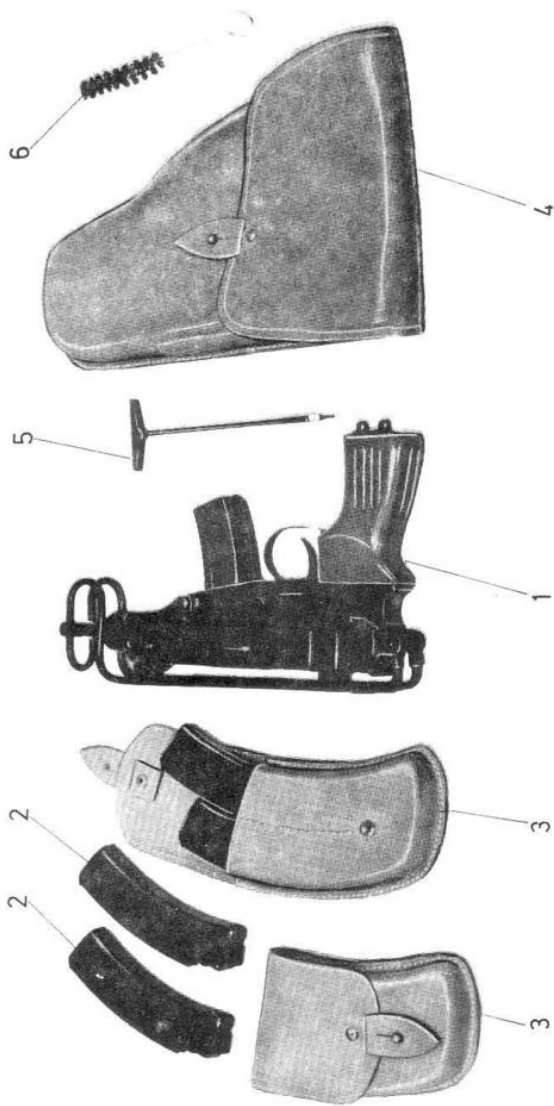
Sl. 3 – Pistolj, automatski 7,65 mm M84 sa priborom:
