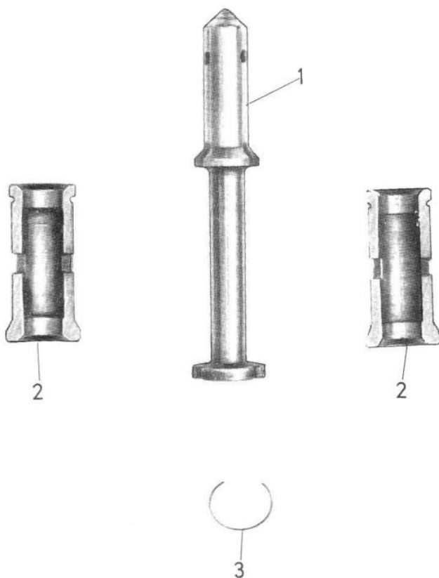
Sl. 20 - Izgled delova rasklopljenog usporivača: 1 - teg usporivača; 2 - protivteg; 3 - prsten protivtega.
