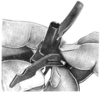
Sl. 87 – Odvajanje poluge automatske paljbe sa osovinom od delova za okidanje
