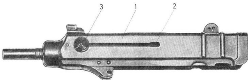
Sl. 26 – Vodica zatvarača sa zatvaračem i opružnim povratnikom (sklop): 1 – vodica zatvarača-sklop; 2 – zatvarač sa opružnim povratnikom (sklop); 3 – hvatač za po- vlačenje zatvarača.
