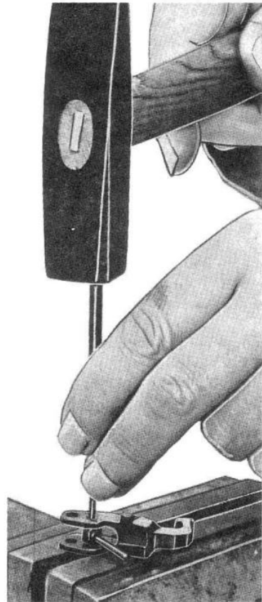
Sl. 91 – Odvajanje osovine vretena udarne opruge od udarače
