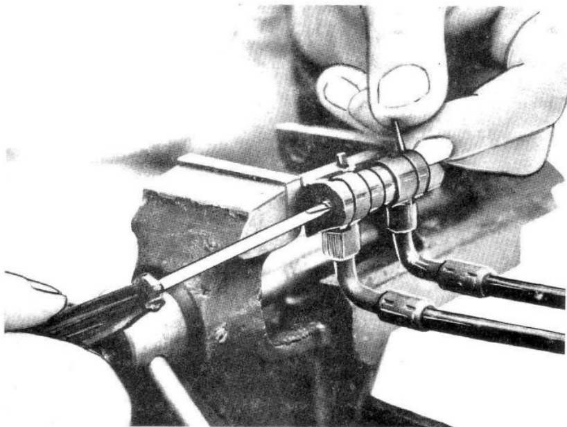
Sl. 107 - Postavljanje utvrdivača osovine kundaka na nosač
