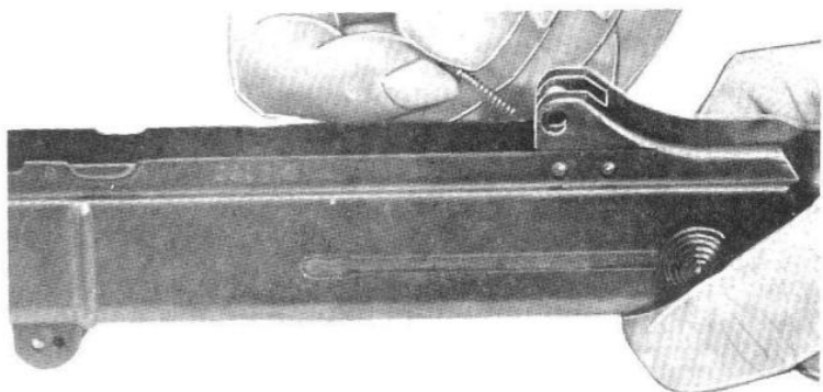
Sl. 60 - Odvajanje utvrdivača osovine vodice zatvarača od sklopa
