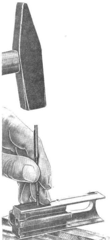
Sl. 68 – Odvajanje osovine igle od zatvarača
