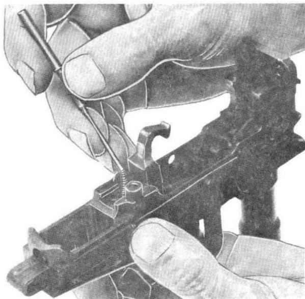
Sl. 75 – Odvajanje opruge utrdne osovine izbacaja
