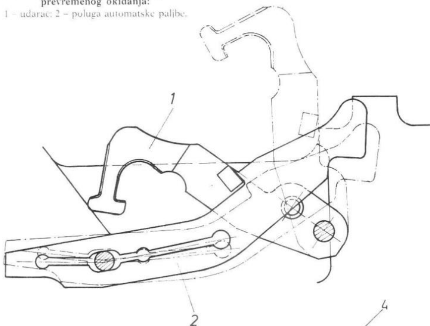
Sl. 10 - Udarač-položaj zuba-osigurača prevremenog okidanja:
