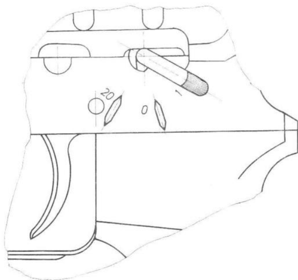
Sl. 8 – Regulator paljbe–kočnica (položaji za izbor paljbe): »1« – jedinačna paljba (poluautomatski rad mehanizma); »0« – ukočen pištolj (blokiran mehanizam za okidanje i zatvarač); »2« – automatska–rafalna paljba (automatski rad mehanizma).
