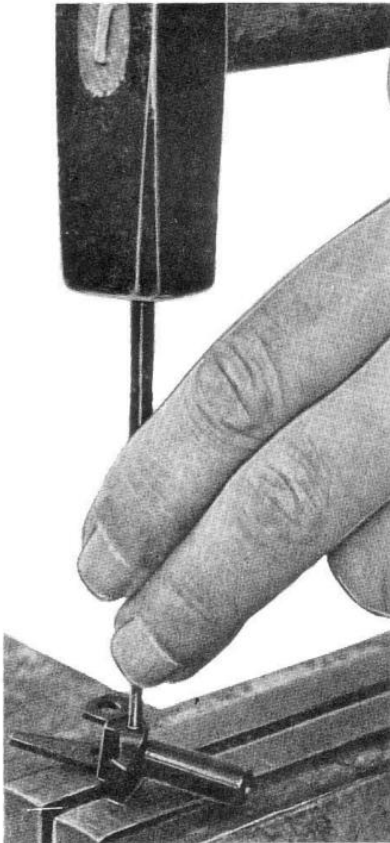
Sl. 90 – Odvajanje osovine vodice udarne opruge od zuba obarače
