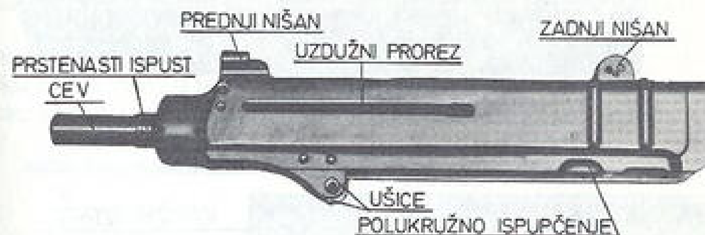
Sl. 2 – Delovi sanduka
