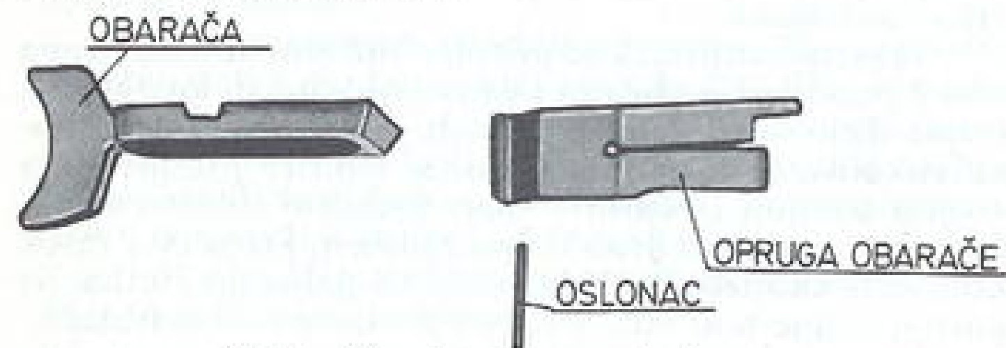
Sl. 11 – Obarača sa oprugom i osloncem
