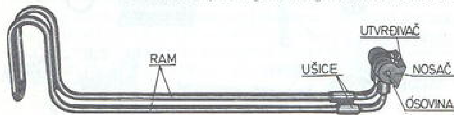
Sl. 14 - Kundak
