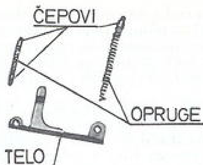
Sl. 12 - Delovi osigurača mehanizma za okidanje
