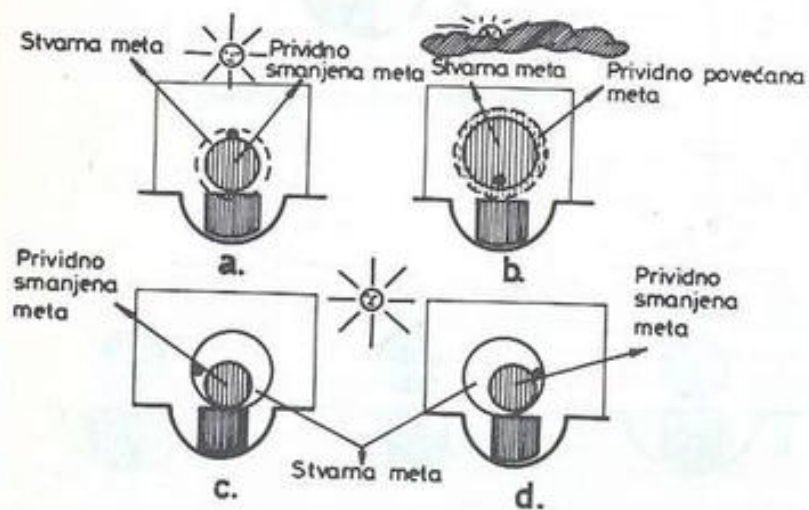
Sl. 36 – Uticaj svetlosti na meti
