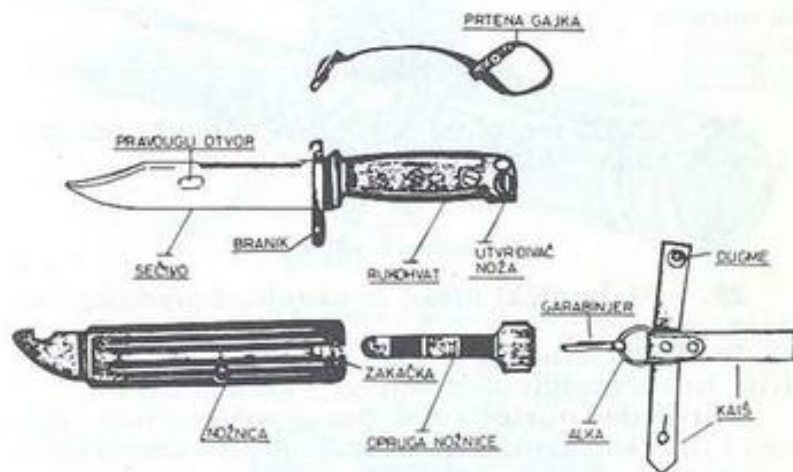
Sl. 13 – Delovi noža sa nožicom
